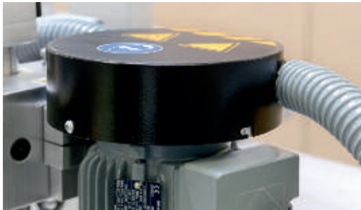
Doppelschleifrad mit grobem (P120) und feinem (P320 oder P400) Schleifband. Alternativ: diamantbeschichtetes Doppelschleifrad mit grober und feiner industrieller Diamantbeschichtung.
